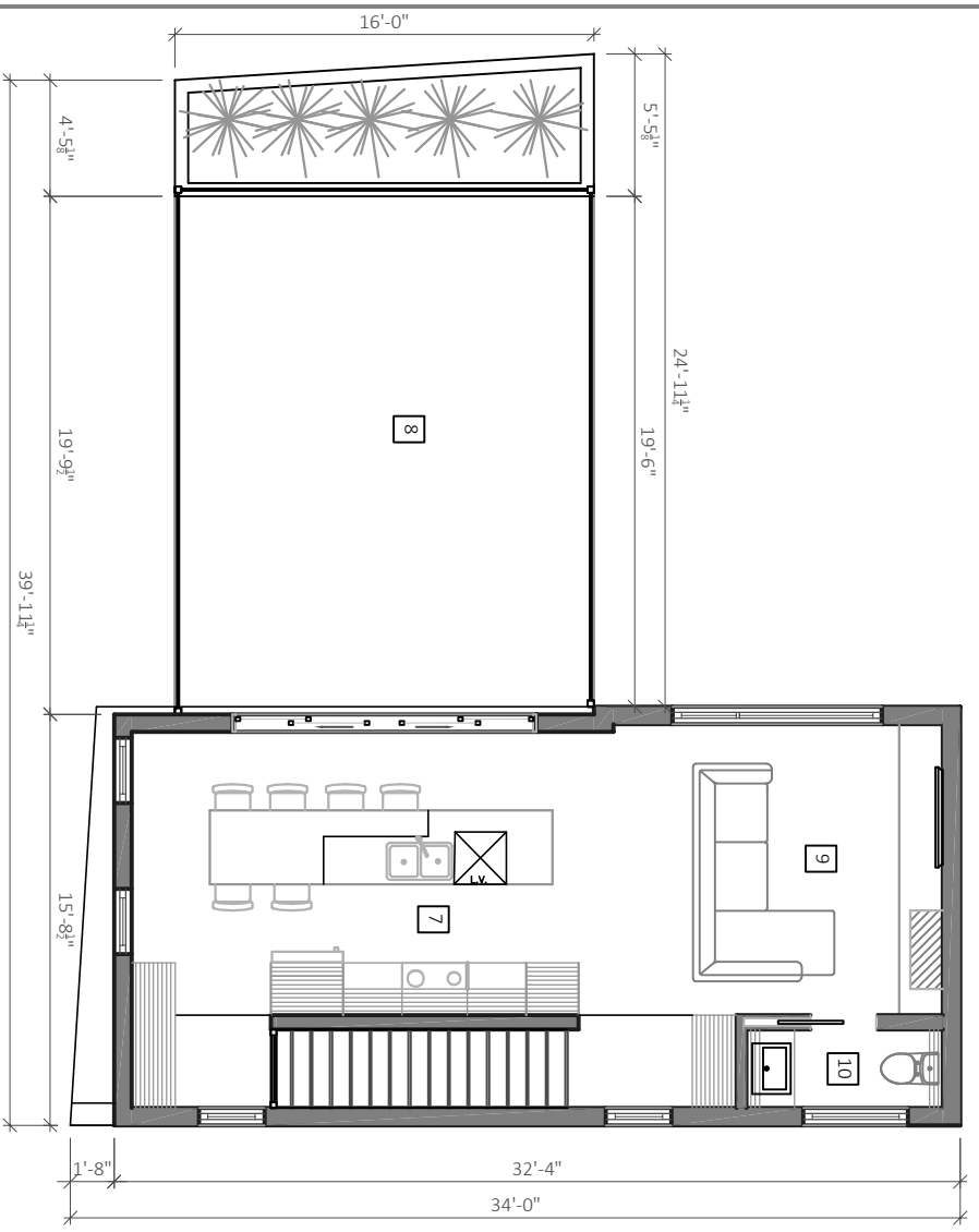
PLAN ÉTAGE
