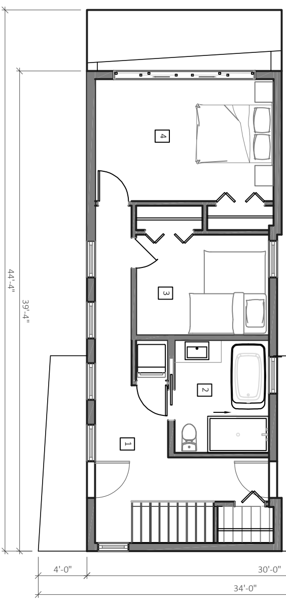
PLAN REZ-DE-CHAUSSE
