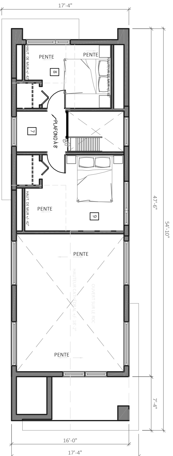
PLAN ÉTAGE
