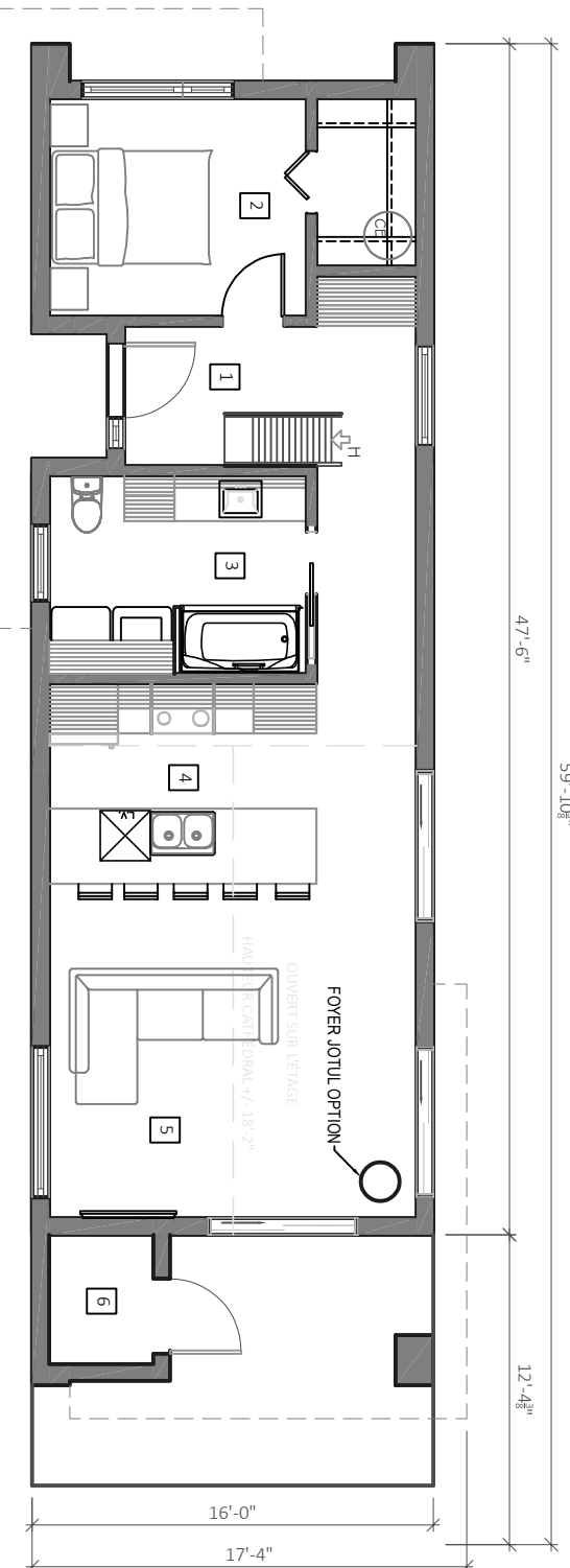
PLAN REZ-DE-CHAUSSE
